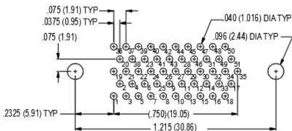
51 SOCKET M83513/32-G
