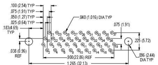
37 SOCKET M83513/31-F
