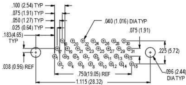
31 SOCKET M83513/31-E
