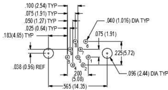
9 PIN M83513/28-A
