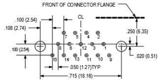
15 SOCKET M83513/13-B
