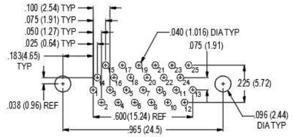
25 SOCKET M83513/31-D
