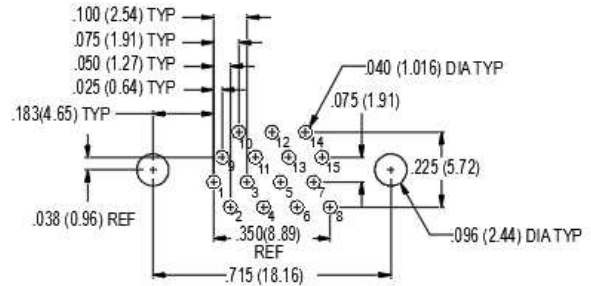
15 SOCKET M83513/31-B
