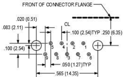
9 SOCKET M83513/13-A
