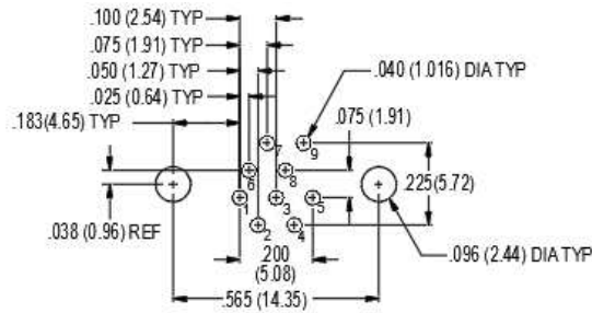
9 SOCKET M83513/31-A
