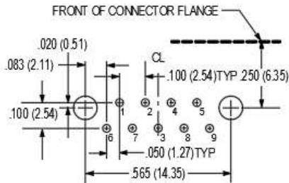
9 PIN M83513/10-A
